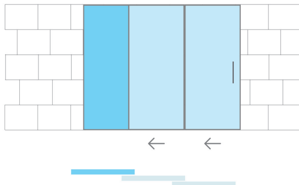
Окачен таван + фикс
