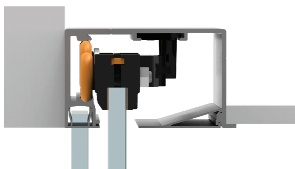
Окачен таван с фиксирано стъкло
