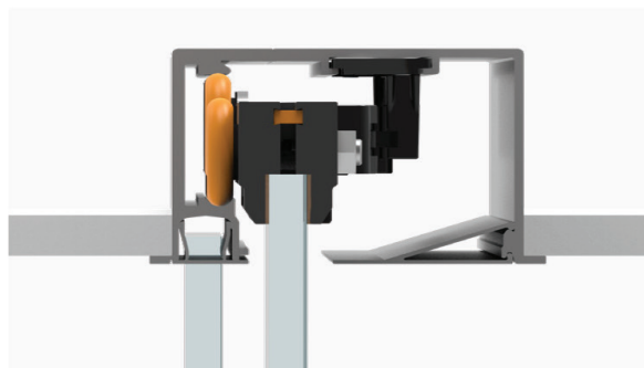
Окачен таван с фиксиран панел
